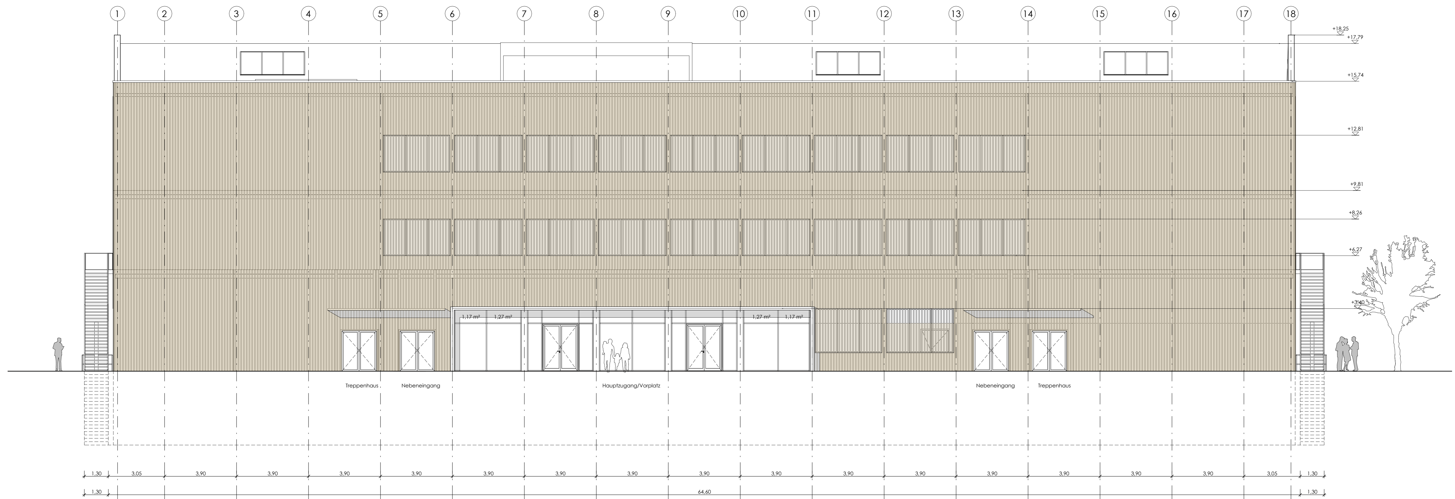
Ansicht Nord
